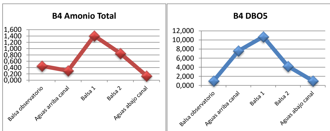
Figuras 7 y 8. Gráfico de resultados para amonio y DBO5 previo a la entrada de agua en la actuación B4.
