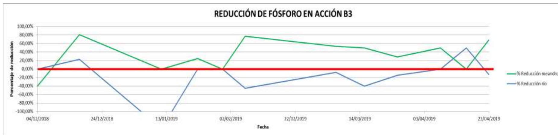
Figura 24. Reducción de fósforo en la acción B3. Porcentaje en meandro y en río.
