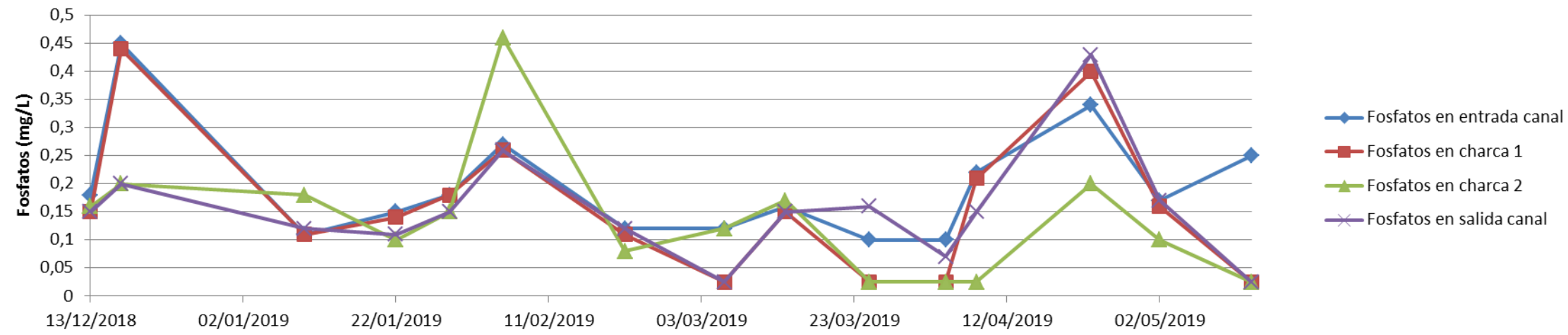
Figura 34. Resultados de control de fosfatos y gráfico de evolución en los puntos de control de la acción B4.
