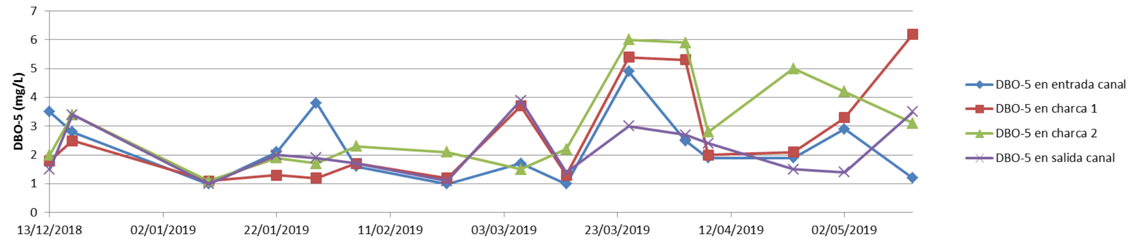
Figura 33. Resultados de control de DBO 5 y gráfico de evolución en los puntos de control de la acción B4.
