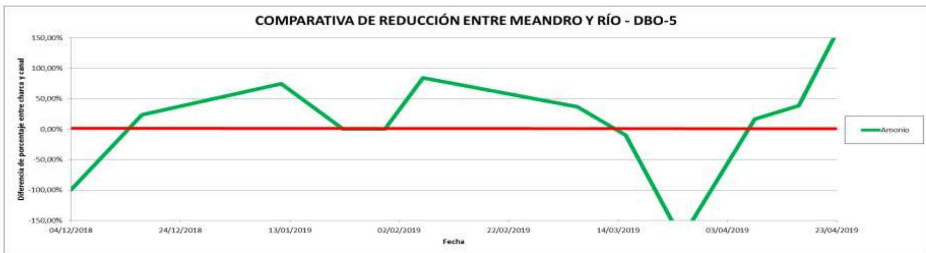
Figura 29. Comparativa de porcentaje de reducción de DBO 5 entre meandro y río.
