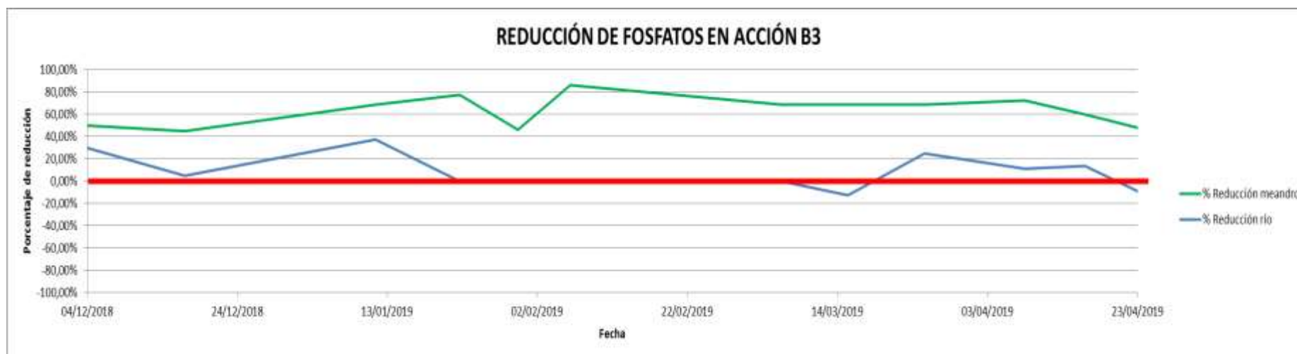
Figura 23. Reducción de fosfatos en la acción B3. Porcentaje en meandro y en río.
