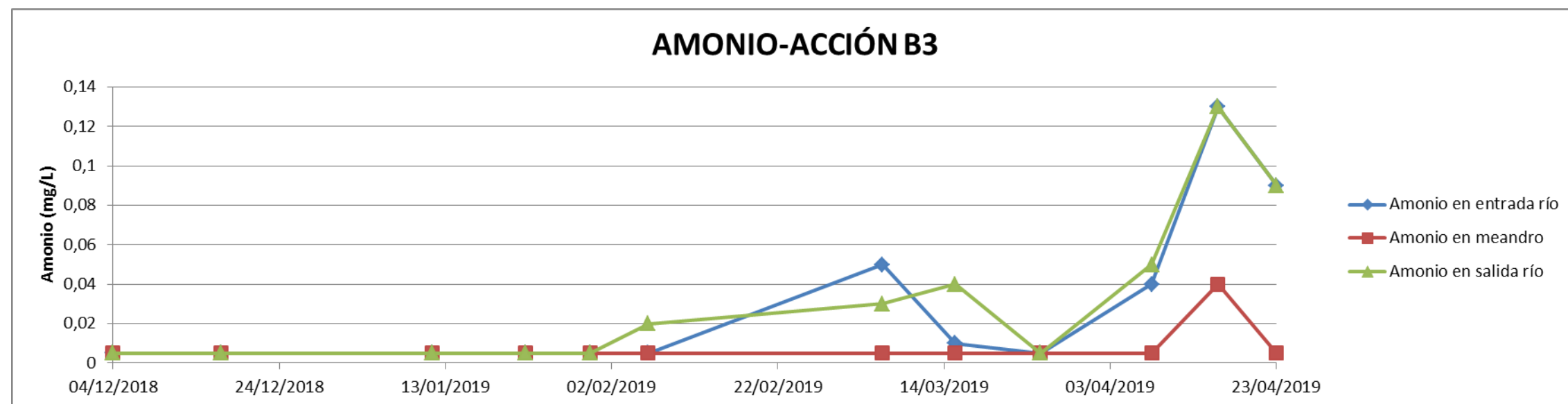
Figura 16. Resultados de control de amonio y gráfico de evolución en los puntos de control de la acción B3.
