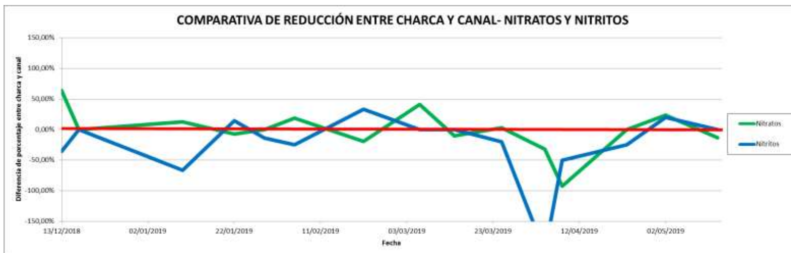
Figura 42. Comparativa de porcentaje de reducción de nitratos y nitritos entre charca y canal.
