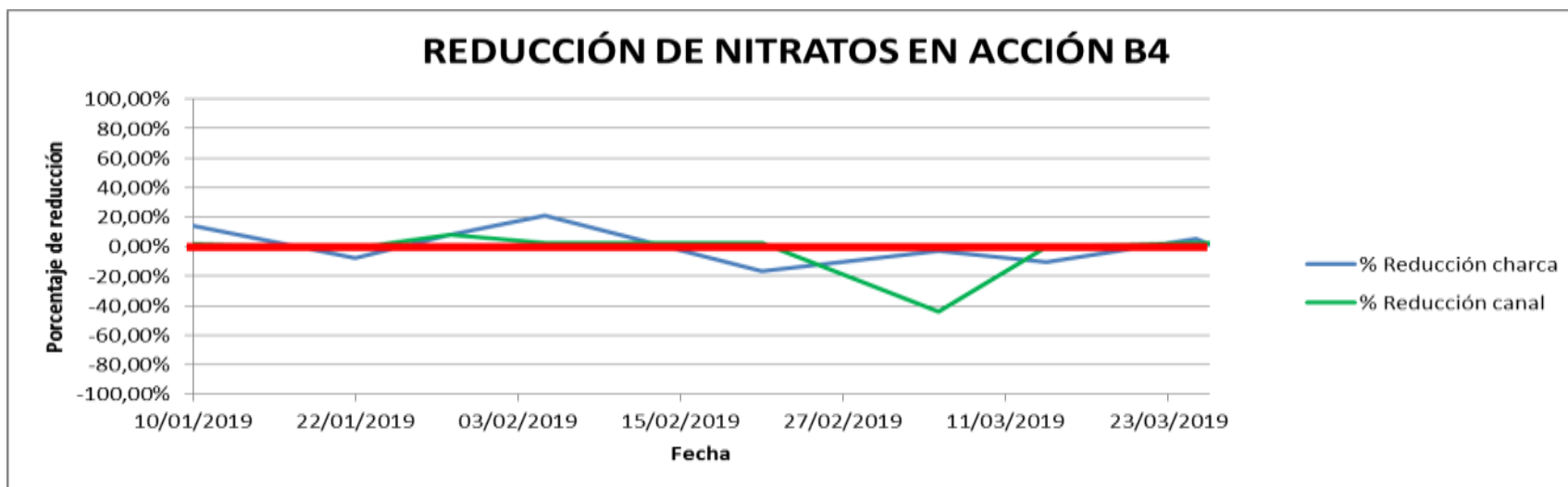
Figura 36. Reducción de nitratos en la acción B4. Porcentaje en charca y en canal.
