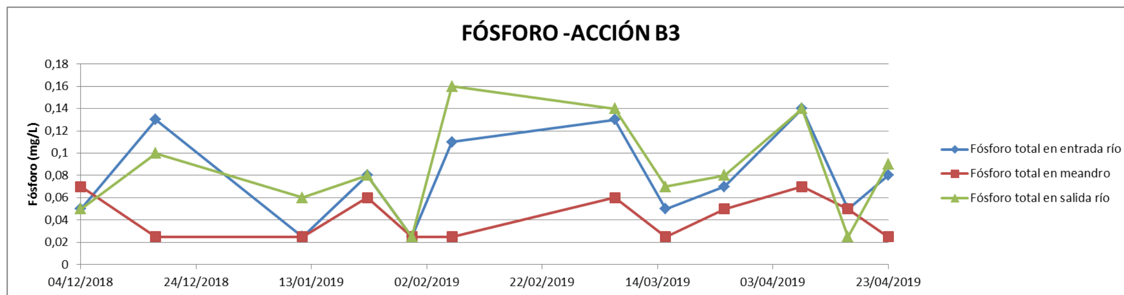
Figura 19. Resultados de control de fósforo y gráfico de evolución en los puntos de control de la acción B3.
