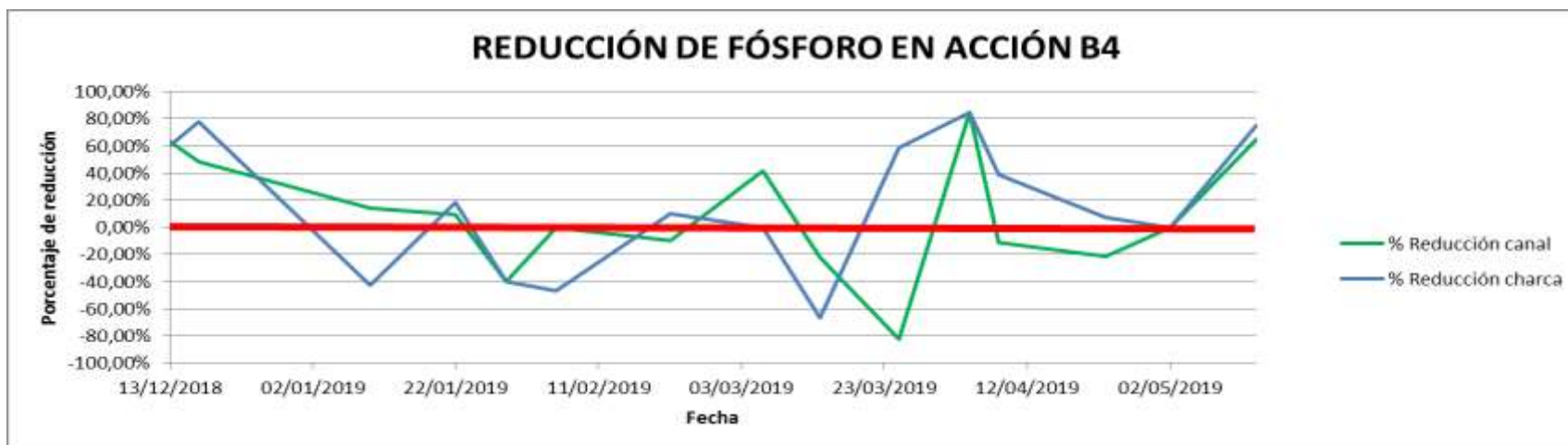
Figura 40. Reducción de fósforo en la acción B4. Porcentaje en charca y en canal.
