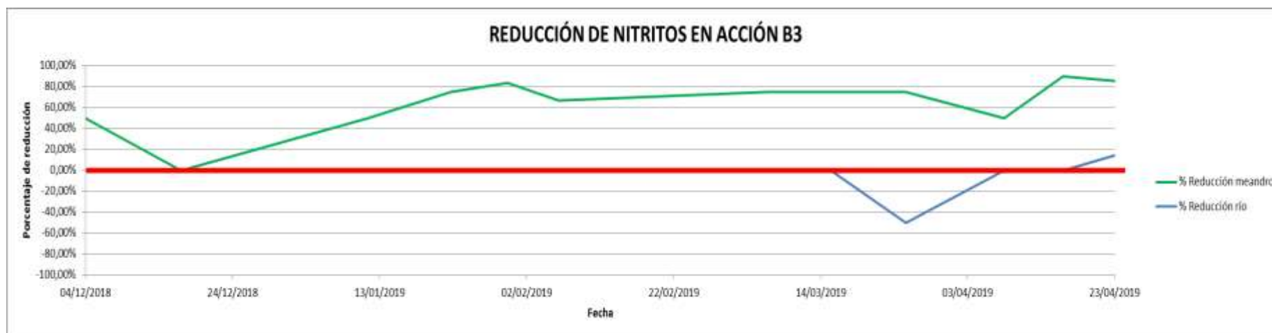
Figura 21. Reducción de nitritos en la acción B3. Porcentaje en meandro y en río.
