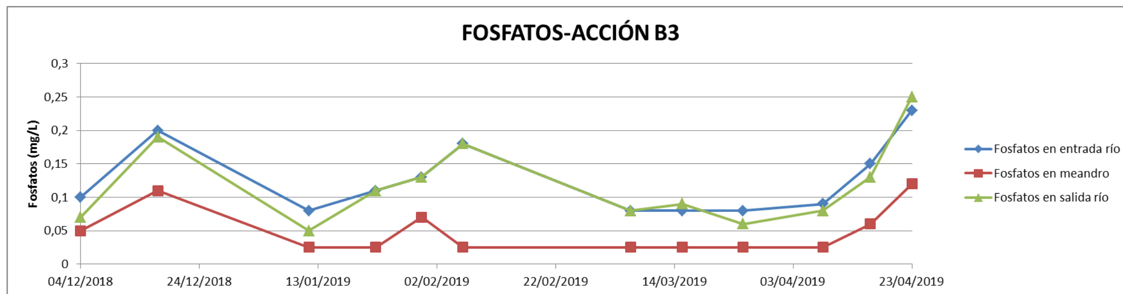
Figura 18. Resultados de control de fosfatos y gráfico de evolución en los puntos de control de la acción B3.
