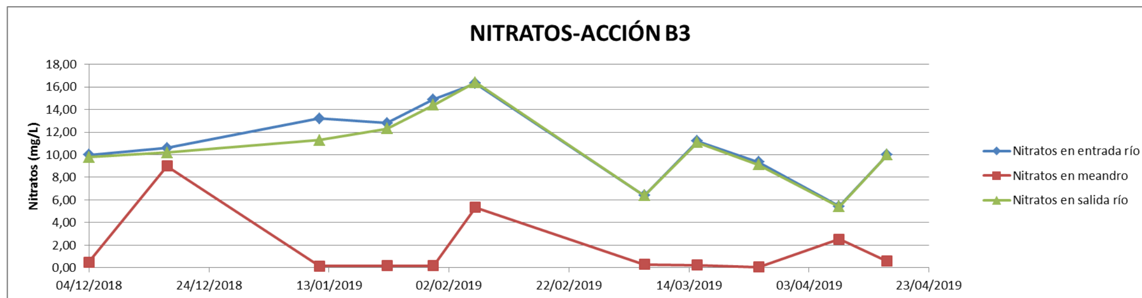
Figura 14. Resultados de control de nitratos y gráfico de evolución en los puntos de control de la acción B3.
