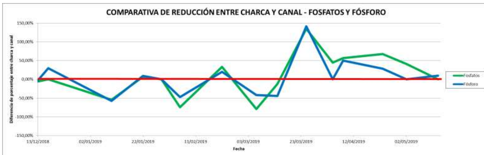
Figura 44. Comparativa de porcentaje de reducción de fosfatos y fósforo entre charca y canal.
