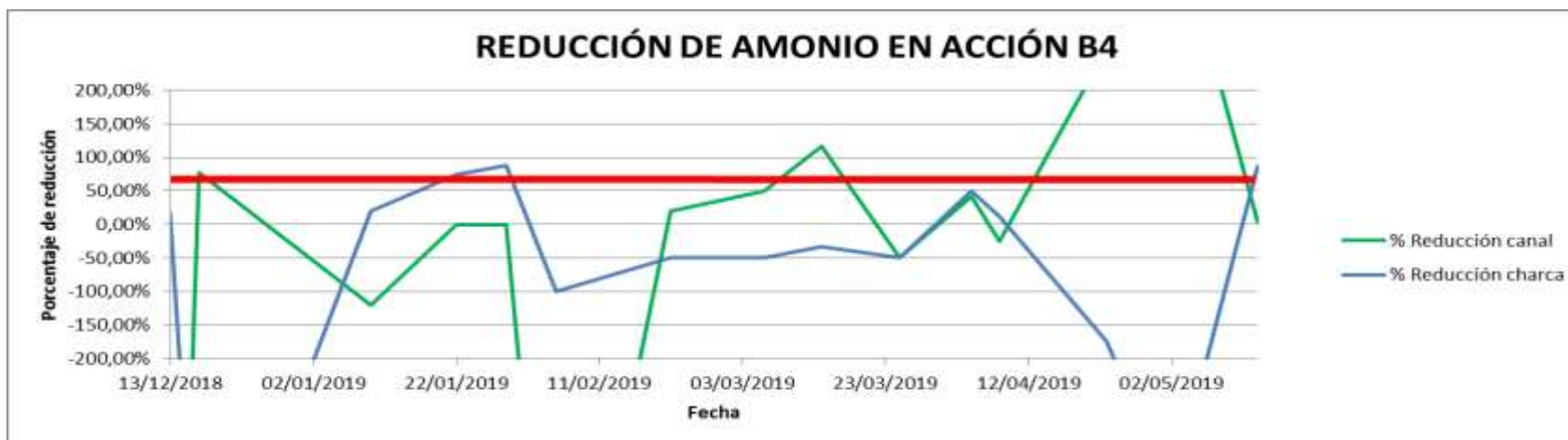
Figura 38. Reducción de amonio en la acción B4. Porcentaje en charca y en canal.
