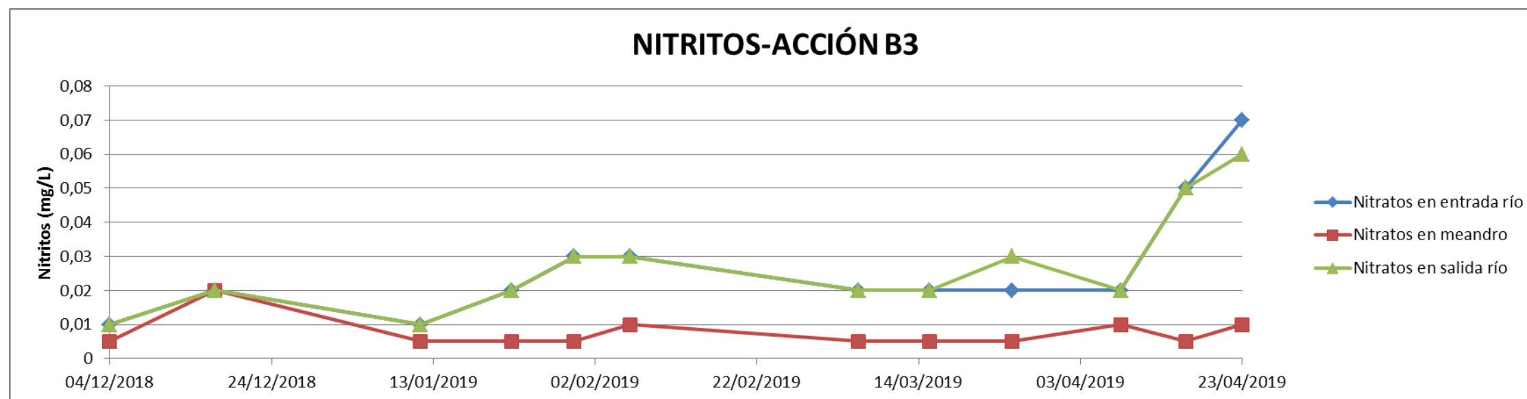
Figura 15. Resultados de control de nitritos y gráfico de evolución en los puntos de control de la acción B3.
