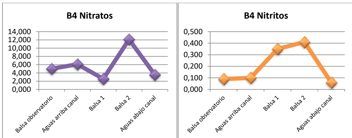
Figuras 11 y 12. Gráfico de resultados para nitratos y nitritos previo a la entrada de agua en la actuación B4.
