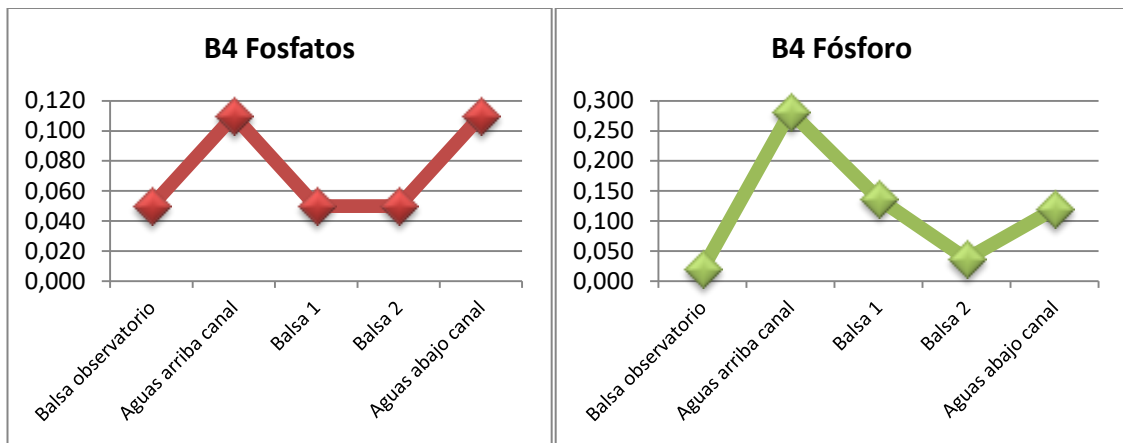
Figuras 9 y 10. Gráfico de resultados para fosfatos y fósforo previo a la entrada de agua en la actuación B4.
