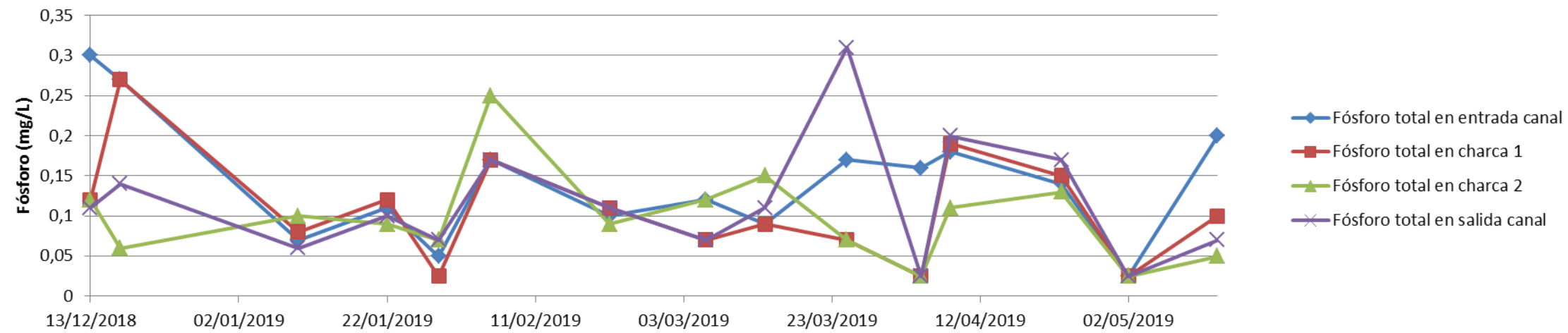
Figura 35. Resultados de control de fósforo y gráfico de evolución en los puntos de control de la acción B4.
