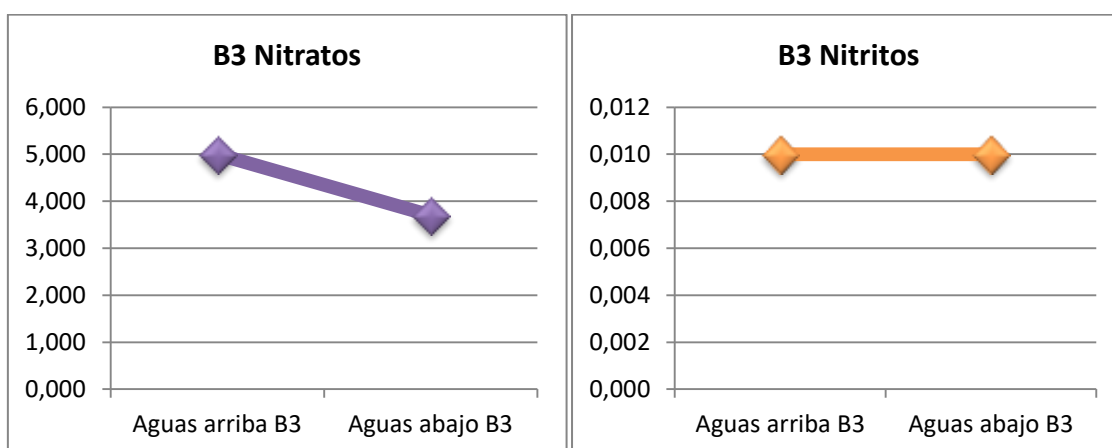
Figuras 5 y 6. Gráfico de resultados para nitratos y nitritos previo a la entrada de agua en la actuación B3.
